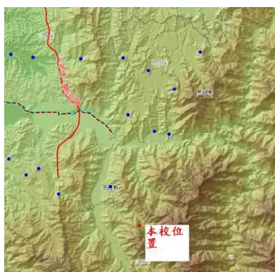
圖 2-2-1、活動斷層圖
